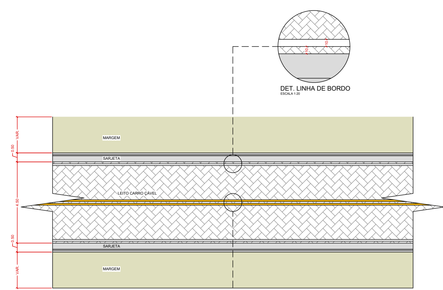
DETALHE SINALIZAÇÃO HORIZONTAL ESCALA 1:100
